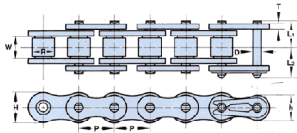
TIPO REMACHADO
