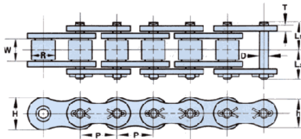
TIPO DESMONTABLE
